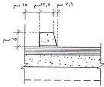
مصدرة مثبتة بالأرضية بمادة الايبوكسي اللاصقة
